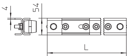
Dimensions
