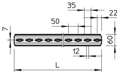
TP-Profil gelocht in der Lieferlänge 3000 mm.
