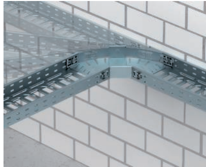
Richtungsänderung durch variablen Bogen Magic Mit dem variablen Bogen Magic Typ RB W... lassen sich stufenlose Richtungsänderungen von 0° - 90° in die Streckenführung einbauen.
