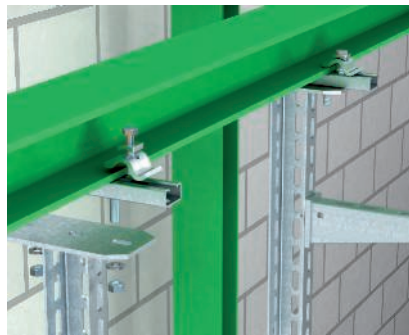
Klemmbefestigung mit zusätzlichem C-Profil Einsatz einer zusätzlichen C-Profilschiene Typ MS bei breiteren Stahlträgern. Trassenverlauf längs zum Stahlträger.
