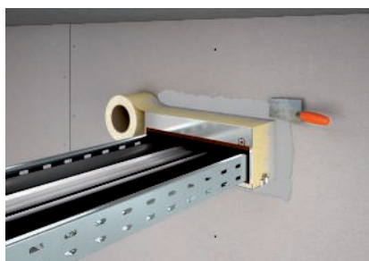
Abkleben und sauberes Einmörteln der Box
