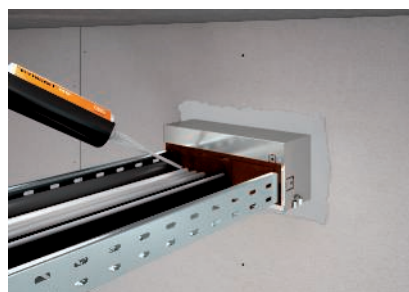
Zwischenräume mit PYROSIT® NG Brandschutzschaum komplett verschließen
