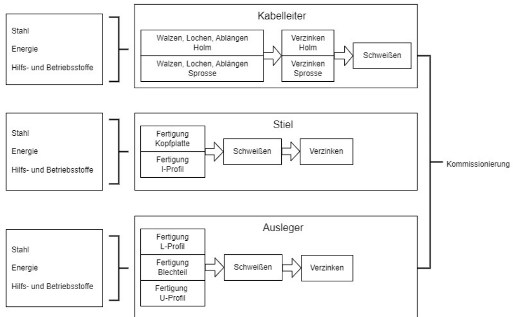
Abbildung 3: Produktherstellung: Kabelleitersystem
