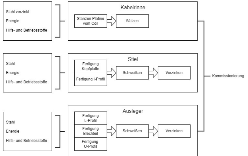
Abbildung 1: Produktherstellung: Kabelrinnensystem
