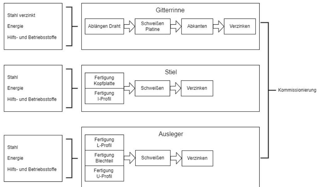
Abbildung 2: Produktherstellung Gitterrinnensystem
