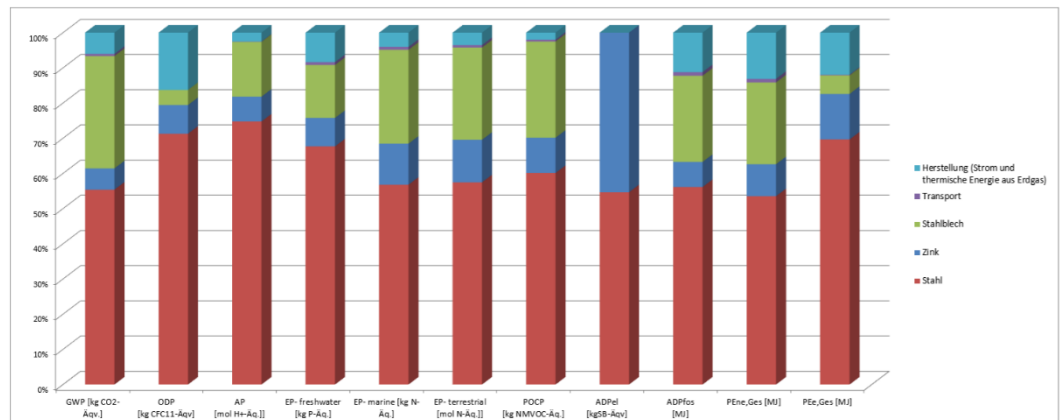
Abbildung 11: Prozentuale Anteile ausgewählter Komponenten der Herstellung und der Transporte im Produktionsstadium anhand ausgewählter Umweltwirkungskategorien (Kabelleitersystem)
