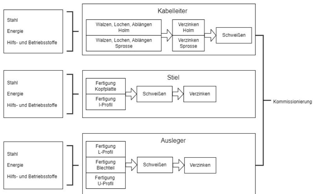
Abbildung 3: Produktherstellung: Kabelleitersystem
