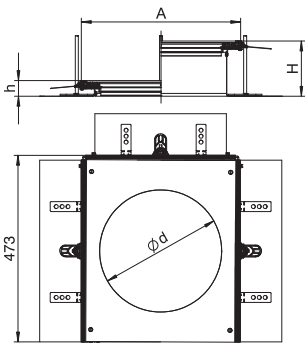
Abmessungen
