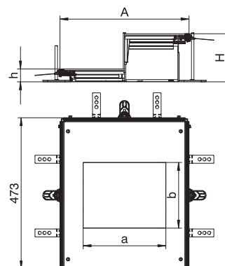
Abmessungen
