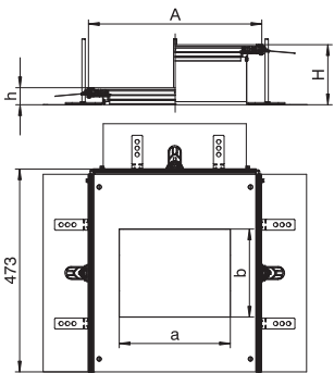
Abmessungen
