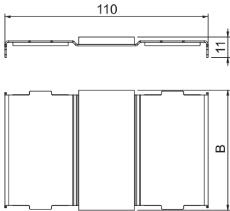
Abmessungen
