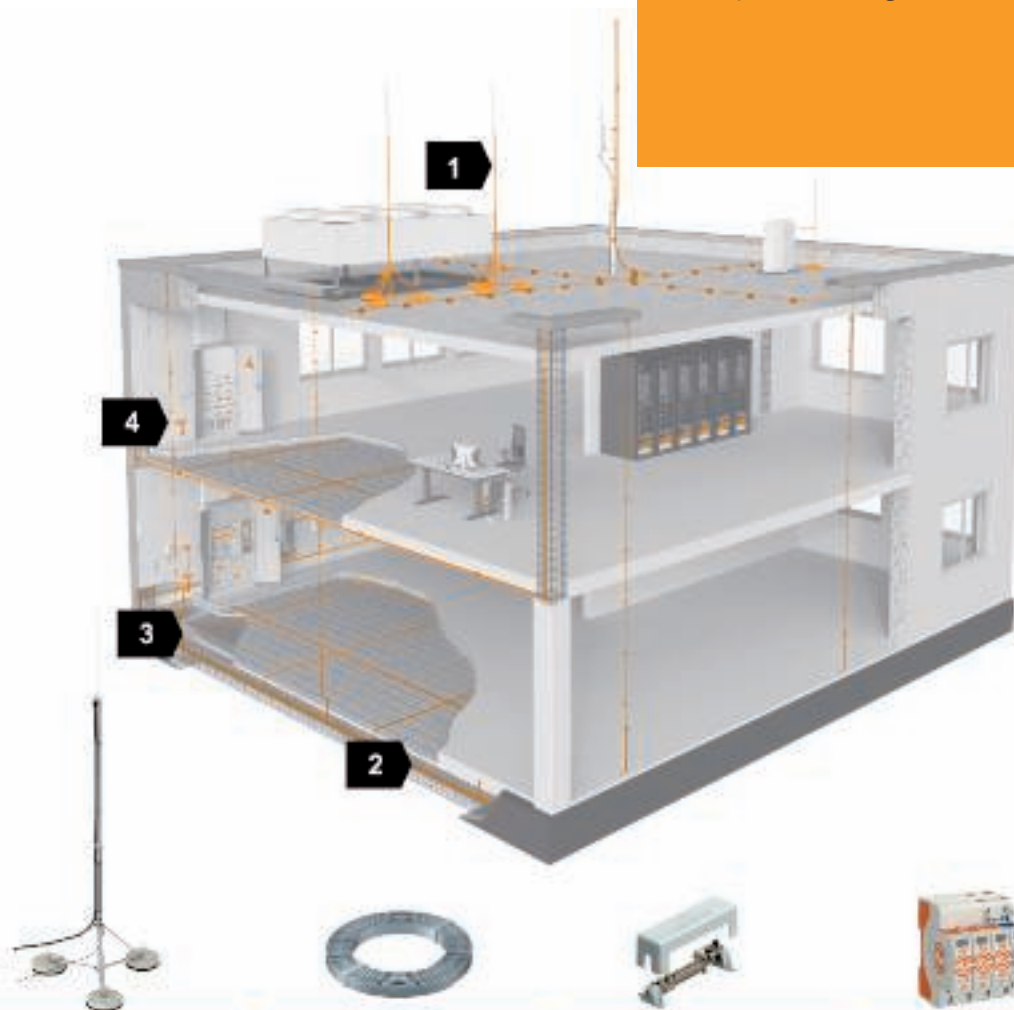
1. Fangeinrichtungs- und Ableitungssysteme
