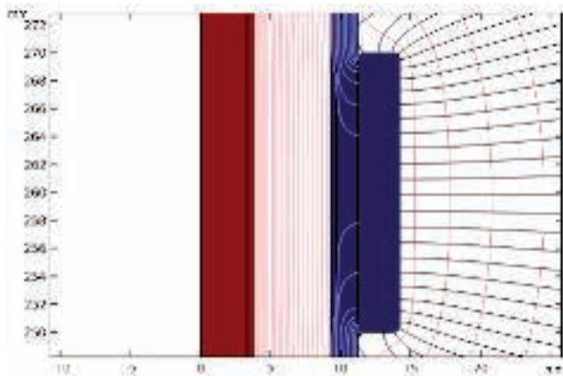
Felddarstellung einer isolierten Ableitung an der ersten Potentialausgleichsklemme während einer Typenprüfung zum Zeitpunkt t = 1,2 \mu\text{s} der angelegten Impulsspannung 1,2/50.
