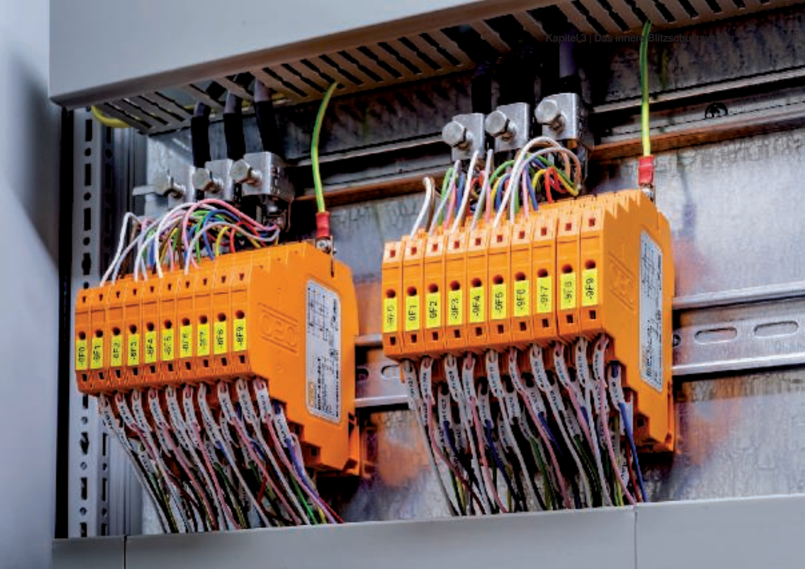
Installationen der MDP-Blitzbarriere im Schaltschrank
