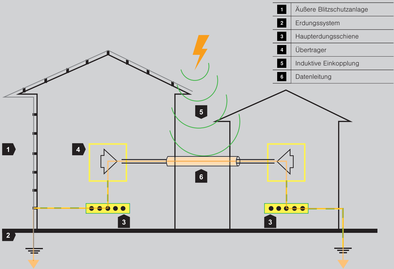
Induktive Einkopplung bei einem Direkteinschlag
