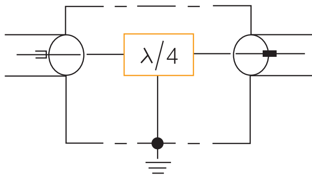
Koaxiales Überspannungsschutzgerät mit Lambda/4 Technologie
