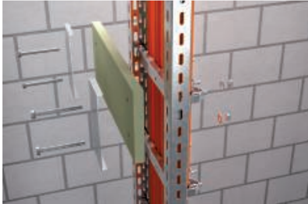
Montieren der Gegenplatte mit Sechskantschrauben an der hängenden Steigtrasse
