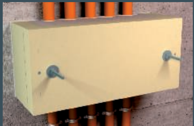
Fertig montierte Zugentlastung mit Mineralwollefüllung
