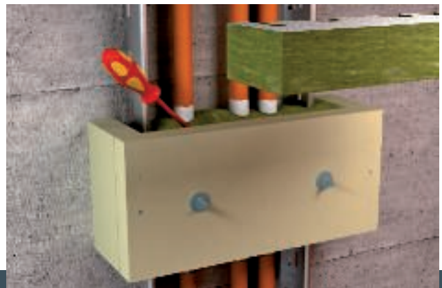
Einbringen der zweiten Mineralfaserplatte oberhalb der Stopfwole
